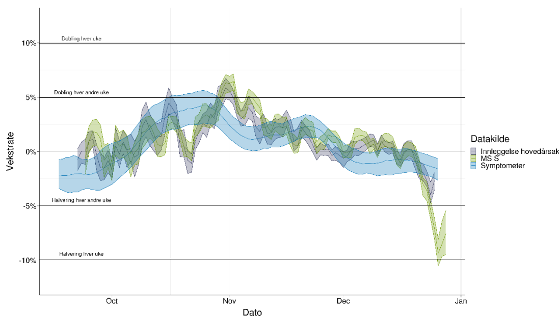
Figur 35. Estimeret vekstrate for nye smittede med covid-19 fra ulike datakilder. En positiv vekstrate indikerer en voksende epidemi og en negativ vekstrate en synkende epidemi. Alle datakildene har styrker og svakheter og må tolkes med varsomhet. Data til og med 31. desember 2023. Kilde: Beredt C19; NPR, MSIS, Symptometer, Folkehelseinstituttet.
